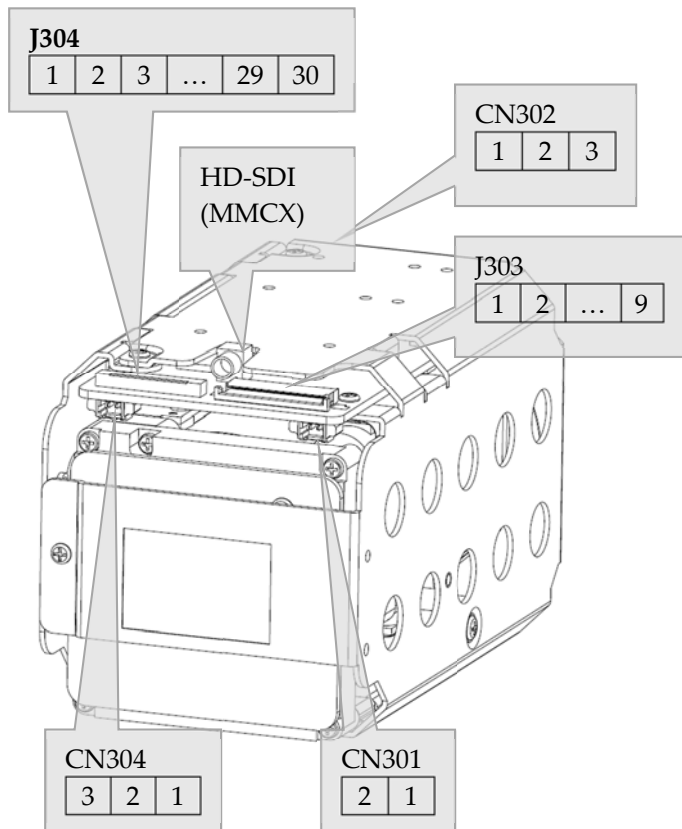
J303 / Molex : 52207-0985
